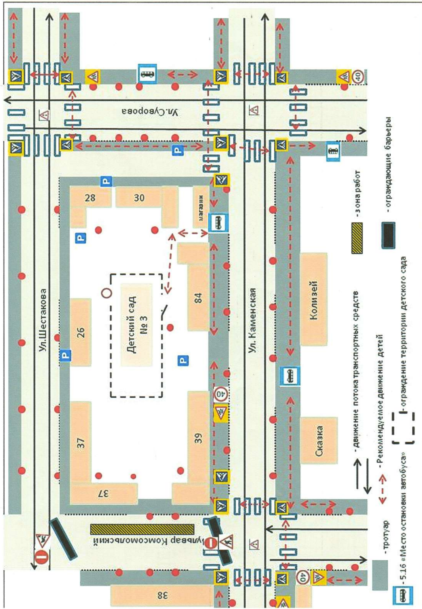
План-схема пути движения транспортных средств и детей при проведении дорожных ремонтно-строительных работ вблизи образовательной организации (1)
